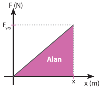
Şekil 4.13: Kuvvet-uzanım grafiği
