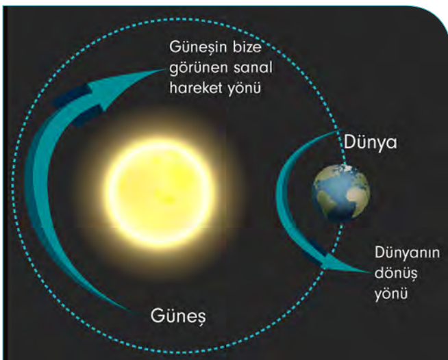
Şekil 3.11: Dünya ve Güneşin dönme hareketi modellenmesi
