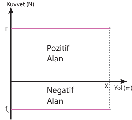
Şekil 4.4: Kuvvet-yol grafiği
