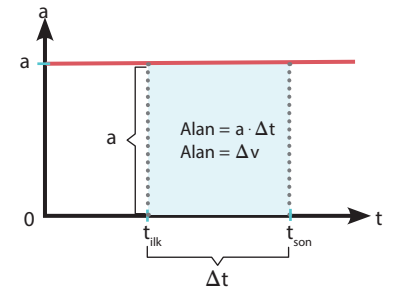
Şekil 3.10: İvme-zaman grafiği
