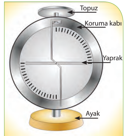
Şekil 6.5: Elektroskopun kısımları
