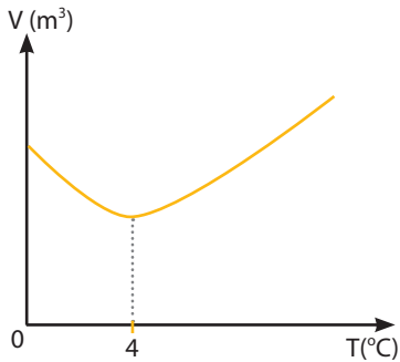
Şekil 5.7: Suyun hacim-sıcaklık değişimi
