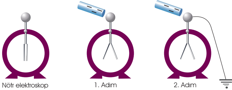
Nötr elektroskop
