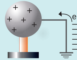
Şekil 6.1.22 (a): Pozitif yüklü kürenin topraklanması
