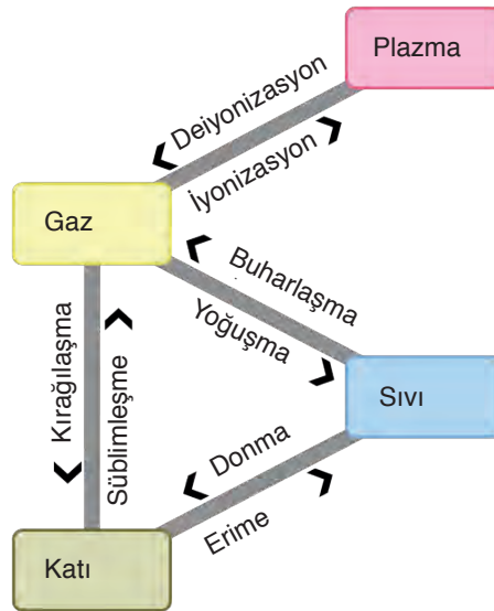
Şekil 5.2.1: Hâl değişimleri
