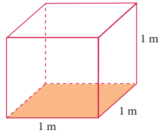
Şekil 2.1.1: Küp
